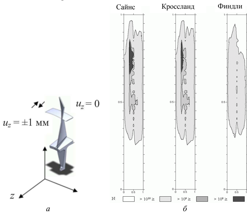
Рис. 4. Схема приложения низкоамплитудных осевых смещений (а) и оценки долговечности титанового диска в зоне концентрации (б)
